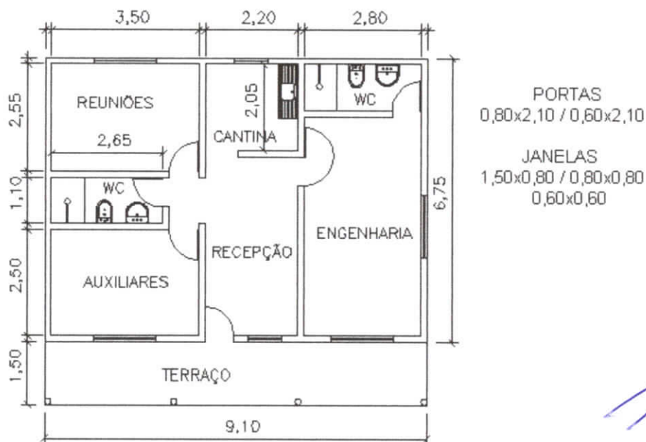
Figura 01: Layout do canteiro de obras - Tipo 01 – Escritório da Fiscalização e Construtora
