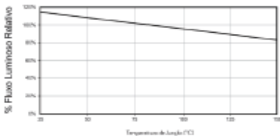
Exemplo de Variação de Fluxo Luminoso em Função da Temperatura de Junção (Tj)
