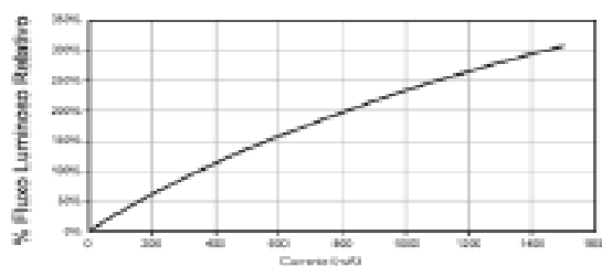
Exemplo de Variação de Fluxo Luminoso em Função de Corrente
