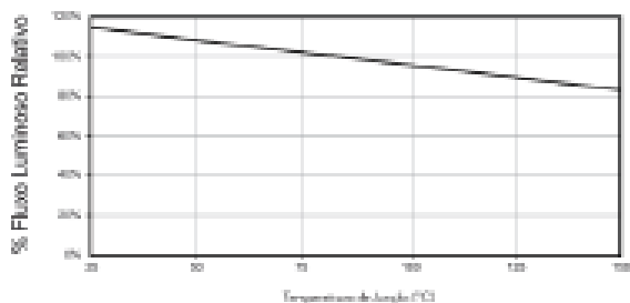
Exemplo de Variação do Fluxo Luminoso em Função da Temperatura de Junção (Tj)
